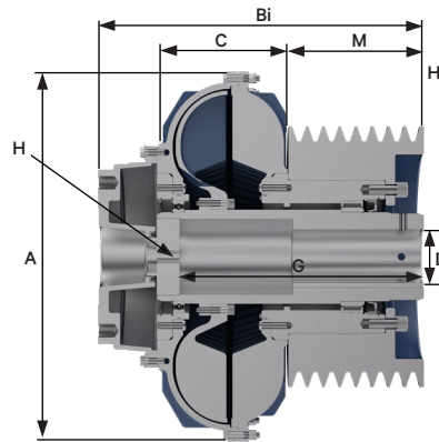
HS.. RVP Delay fill type size 8-12
